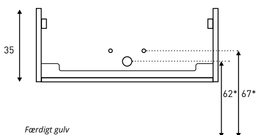
Centerafstand vand og afløb TOPDECK 60 / 70 / 80 / 90 / 100 / 120 / 140 / 180
