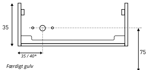
Centerafstand vand og afløb FAKTOR VASK VENSTRE 100 / 120 / 140 / 160 (flad vandlås medleveres)
