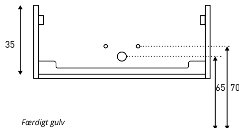
Centerafstand vand og afløb TABLET 90 / 100 / 120 / 140
